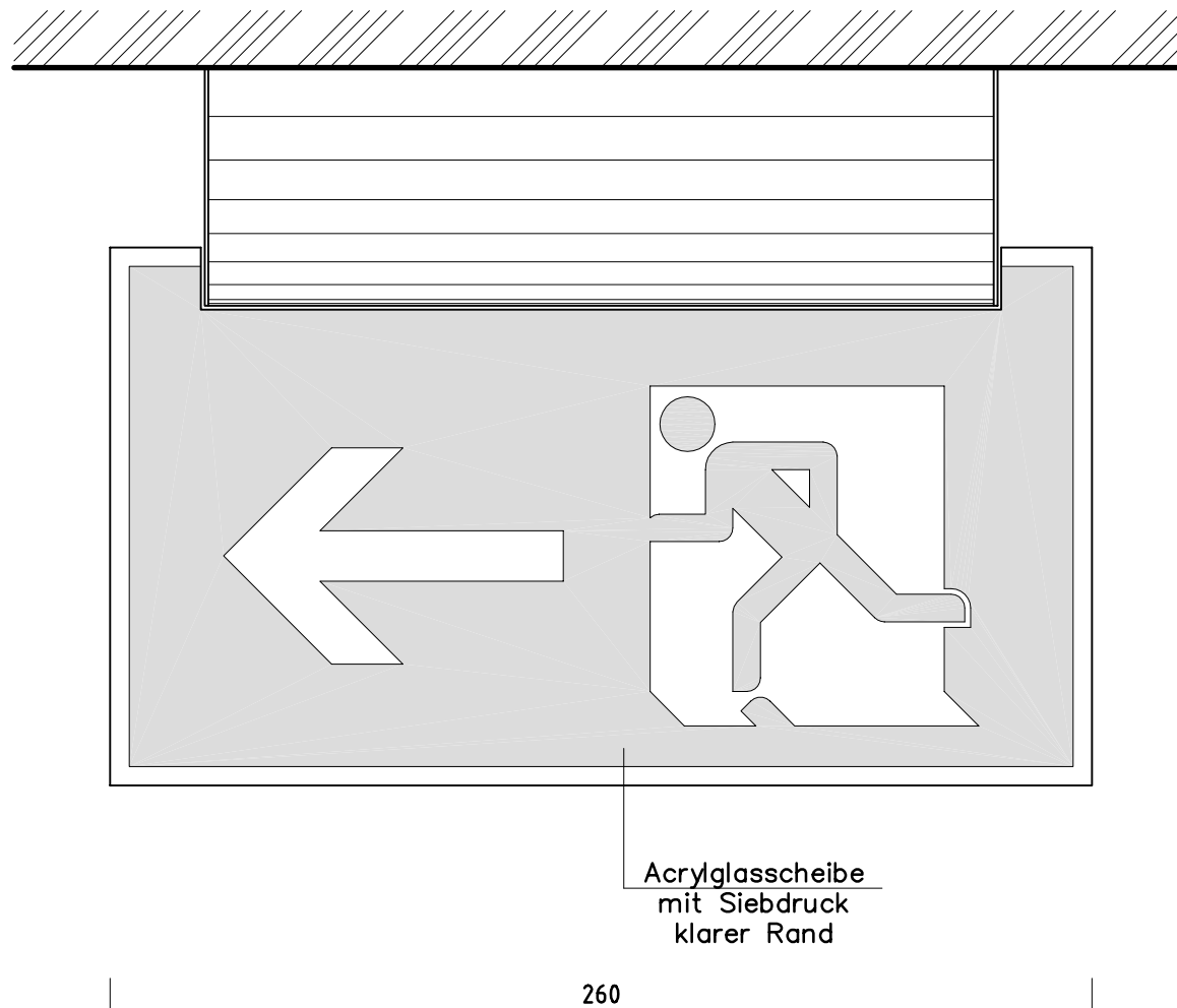
Vorderansicht Deckenaufbau
